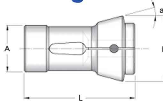
DIN 6343 Single Cone
